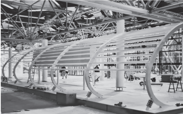
Estructura metàl·lica per a un estant de cotxes en una fira europea, estudiada i feta al taller d'en Joan Tallada.
