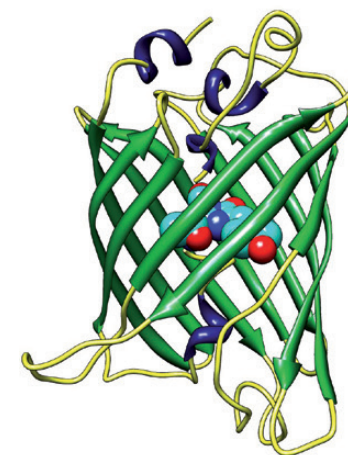
Model molecular de la proteïna GFP
