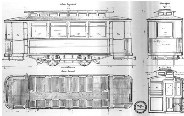
Plànols del tramvia entre Montgat i Tiana, que hauria estat el mateix que per al Masnou.
