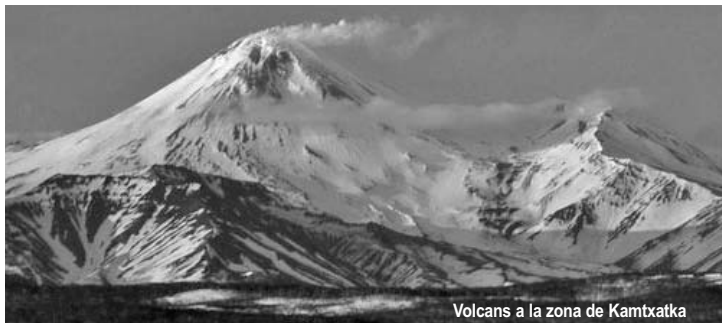
Volcans a la zona de Kamtxatka
